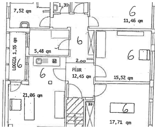
Grundriss Wohnung
