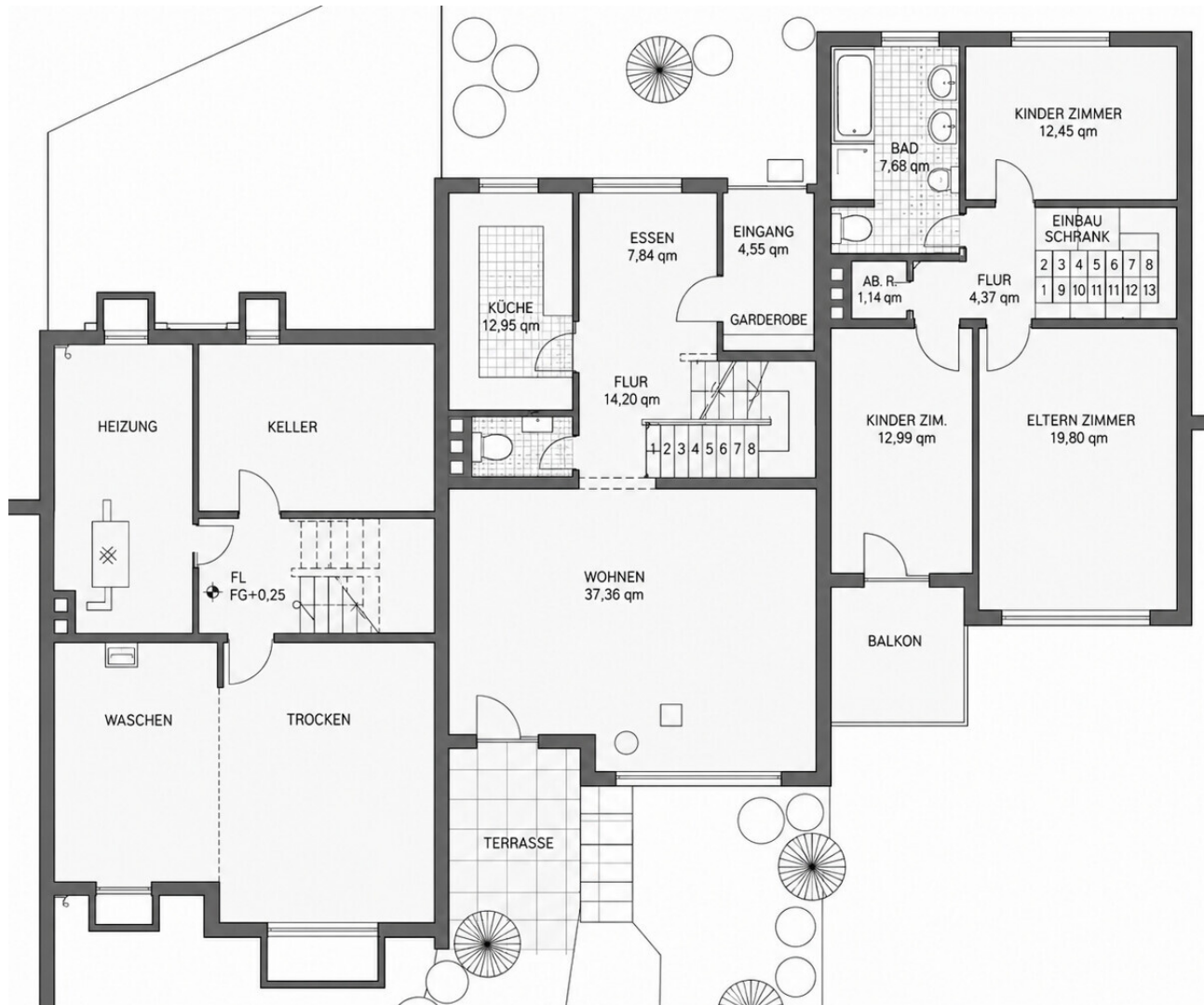
Detaillierter Grundriss
